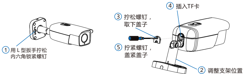
带支架型号TF卡安装
